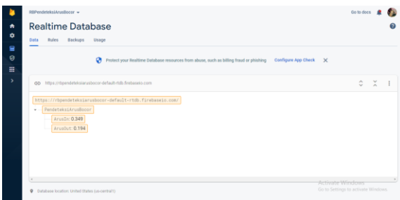
Gambar 11. Tampilan Firebase Pada Beban 45 Watt
