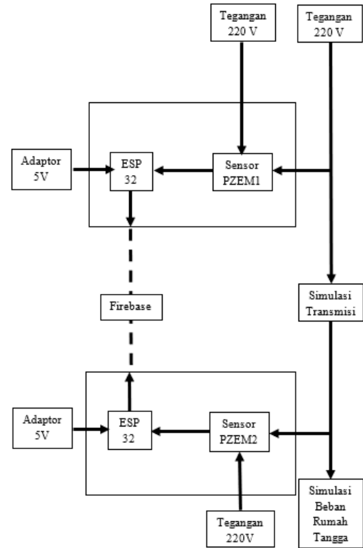
Gambar 1. Diagram Blok Alat
