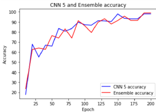
Gambar 3. Grafik perbandingan akurasi CNN 5 dengan ensemble CNN.
