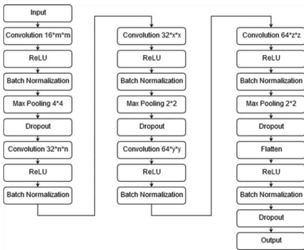
Gambar 1. Arsitektur CNN yang digunakan
