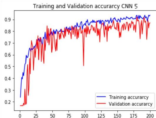
Gambar 2. Grafik perubahan akurasi terhadap jumlah epoch pada data train dan validasi
