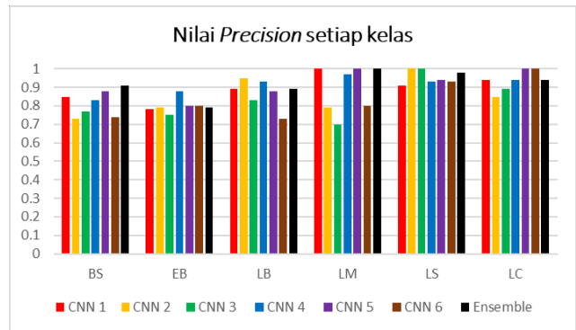
Gambar 5. Hasil precision untuk setiap kelas dengan menggunakan 6 model CNN dan ensemble CNN.
