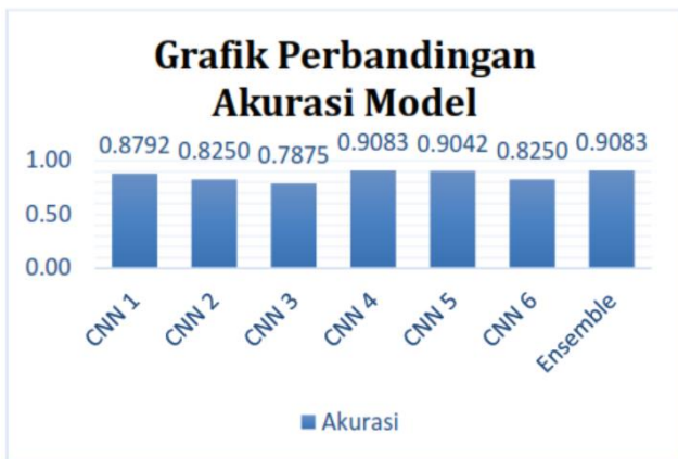
Gambar 4. Perbandingan akurasi model hasil training menggunakan data test.
