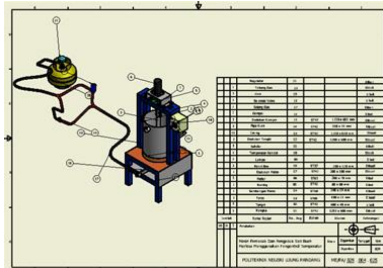
Gambar 1. Desain Mesin Pemasak dan Pengaduk Sari Buah Markisa
