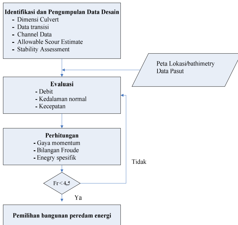
Gambar 3. Diagram Alir Pemilihan bangunan peredam energi
