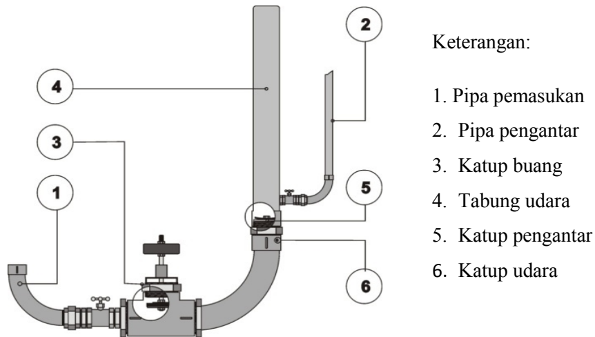
Gambar 5. Desain pompa hidram
