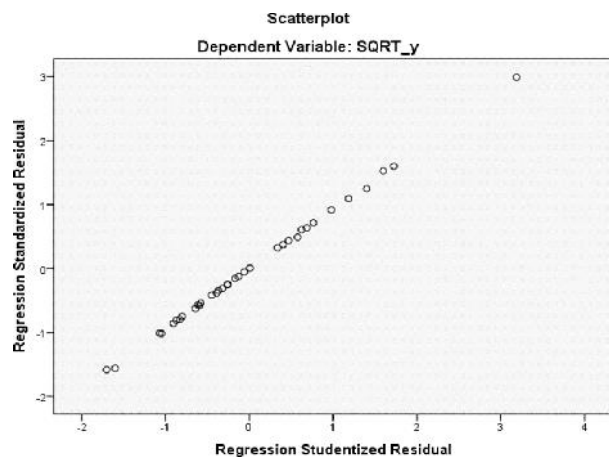
Gambar 2 Grafik Scatterplot
