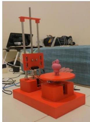
Gambar 2. Mesin 3D Scanner Menggunakan Sensor Jarak Infrared
