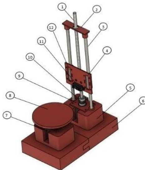
Gambar 1. Desain 3D Scanner Menggunakan Sensor Jarak Infrared
