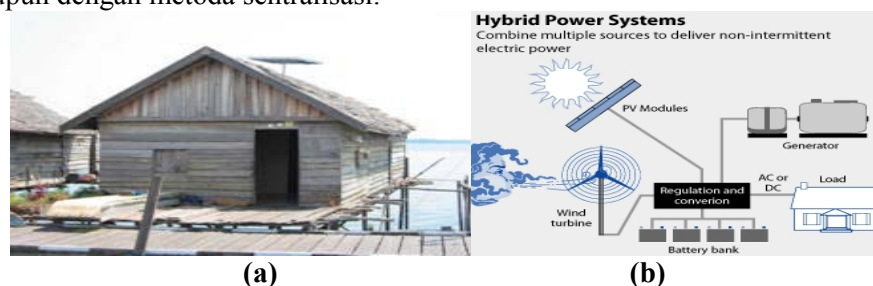
Gambar 1. (a) PLTS Stand Alone (b) PLTS Hybrid dengan Generator dan Wind Sumber : http://www.azetsurya.com/info.php
