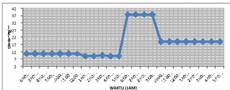
Gambar 5. Kurva Beban Harian Pada Pulau Bahuluang
