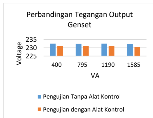
Gambar 7. Grafik Perbandingan Hasil Pengukuran Tegangan
