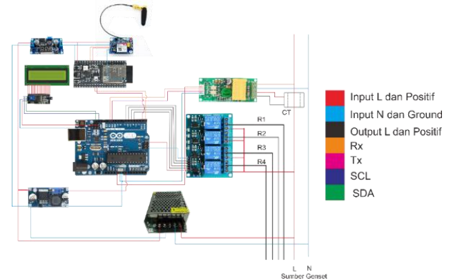
Gambar 4. Tampilan Rangkaian Kontrol Alat
