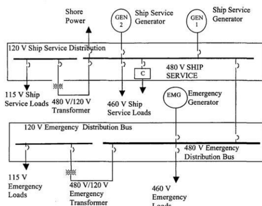
Gambar 1. Diagram Listrik Satu Garis - Pembangkitan dan Distribusi Tenaga Layanan Kapal dengan Dua Generator Layanan Kapal dan Satu Generator Darurat [5] Pada gambar 1 nampak desain terdiri dari satu switchboard layanan kapal dan dua generator layanan kapal. Switchboard darurat dengan satu generator darurat.
