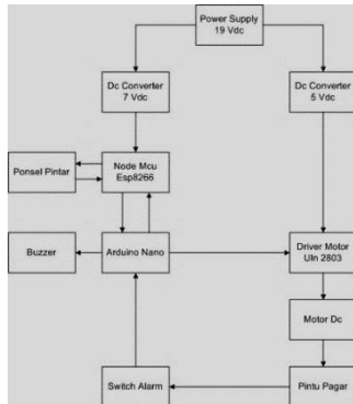
Gambar 6 Rangkaian Perangkat Keras
