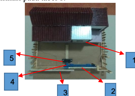
Gambar 9 Hasil Perancangan Rancang Bangun Pintu Pagar Otomatis
