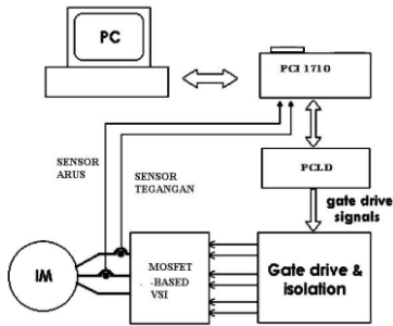
Gambar 3. Blok diagram pemodelan sistem
