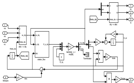
Gambar 4. Model Motor Induksi 3 fasa
