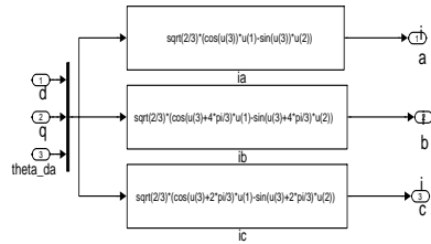
Gambar 7. Transformasi besaran sumbu dq ke abc
