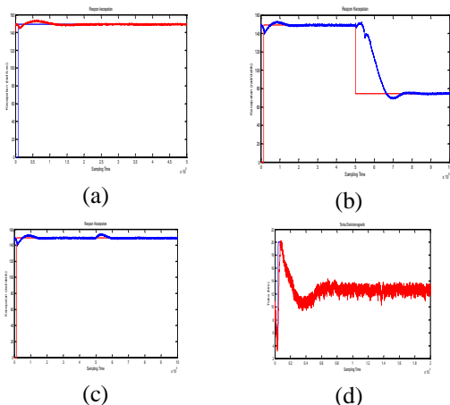
Gambar 10. (a) Putaran motor induksi pada saat start; (b) Putaran pada saat referensi turun 50%; (c) Putaran pada saat beban turun 50%; (d) Torka elektromagnetik motor pada saat start
