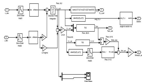
Gambar 8. Estimator flux, torka , putaran dan sudut
