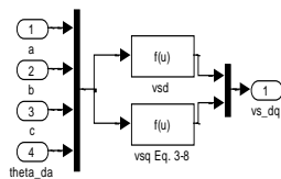
Gambar 6. Transformasi besaran sumbu abc ke dq
