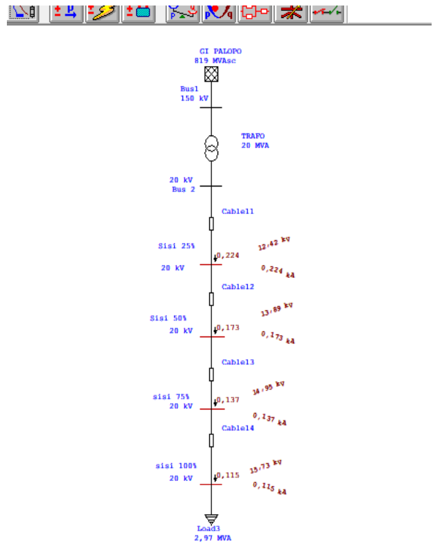
Gambar 21. hasil gambar hubung singkat simulasi menggunakan Etap 12.6.0
