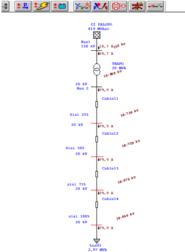
Gambar 20. hasil gambar aliran daya simulasi menggunakan Etap 12.6.0
