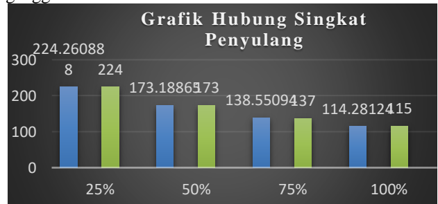
Gambar 24. hasil grafik hubung singkat berdasarkan perhitungan dan simulasi
