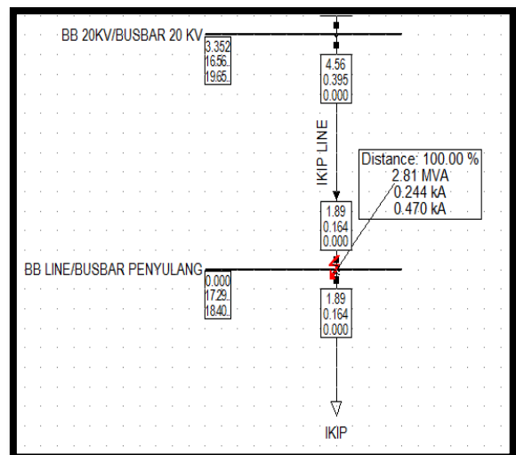
Gambar 8. Simulasi Hubung Singkat 1 Fasa ke Tanah
