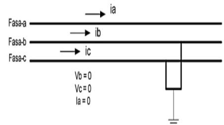
Gambar 3.. Gangguan hubung singkat 2 fasa ke tanah (Sumber : Studi Perencanaan Kordinasi Literatur, Mardensyah)
