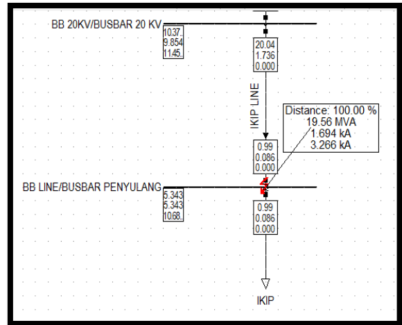
Gambar 5. Simulasi Hubung Singkat 2 Fasa
