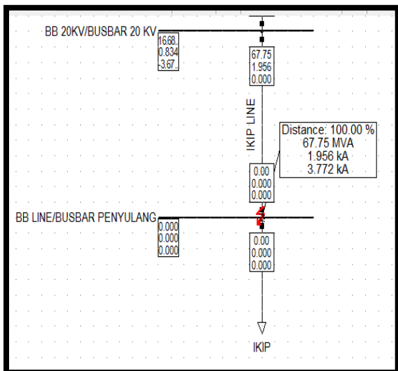
Gambar 7. Simulasi Hubung Singkat 3 Fasa
