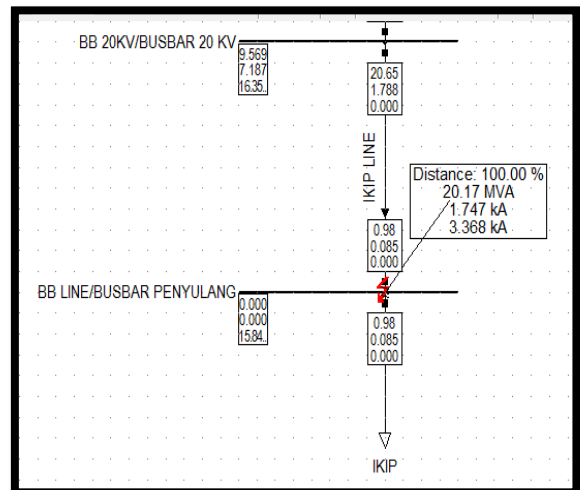
Gambar 6. Simulasi Hubung Singkat 2 Fasa ke Tanah
